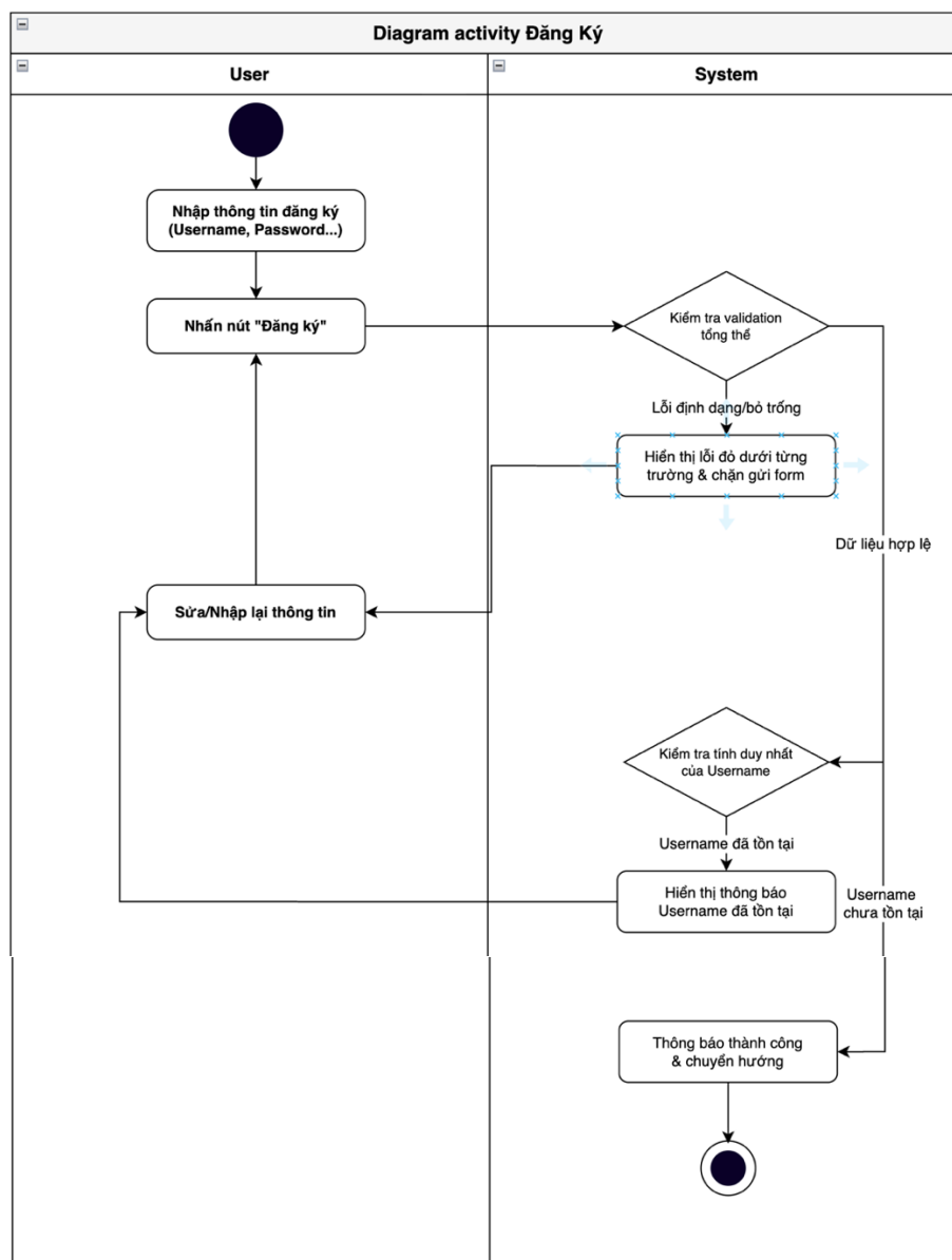
Hình 2: Activity Diagram
