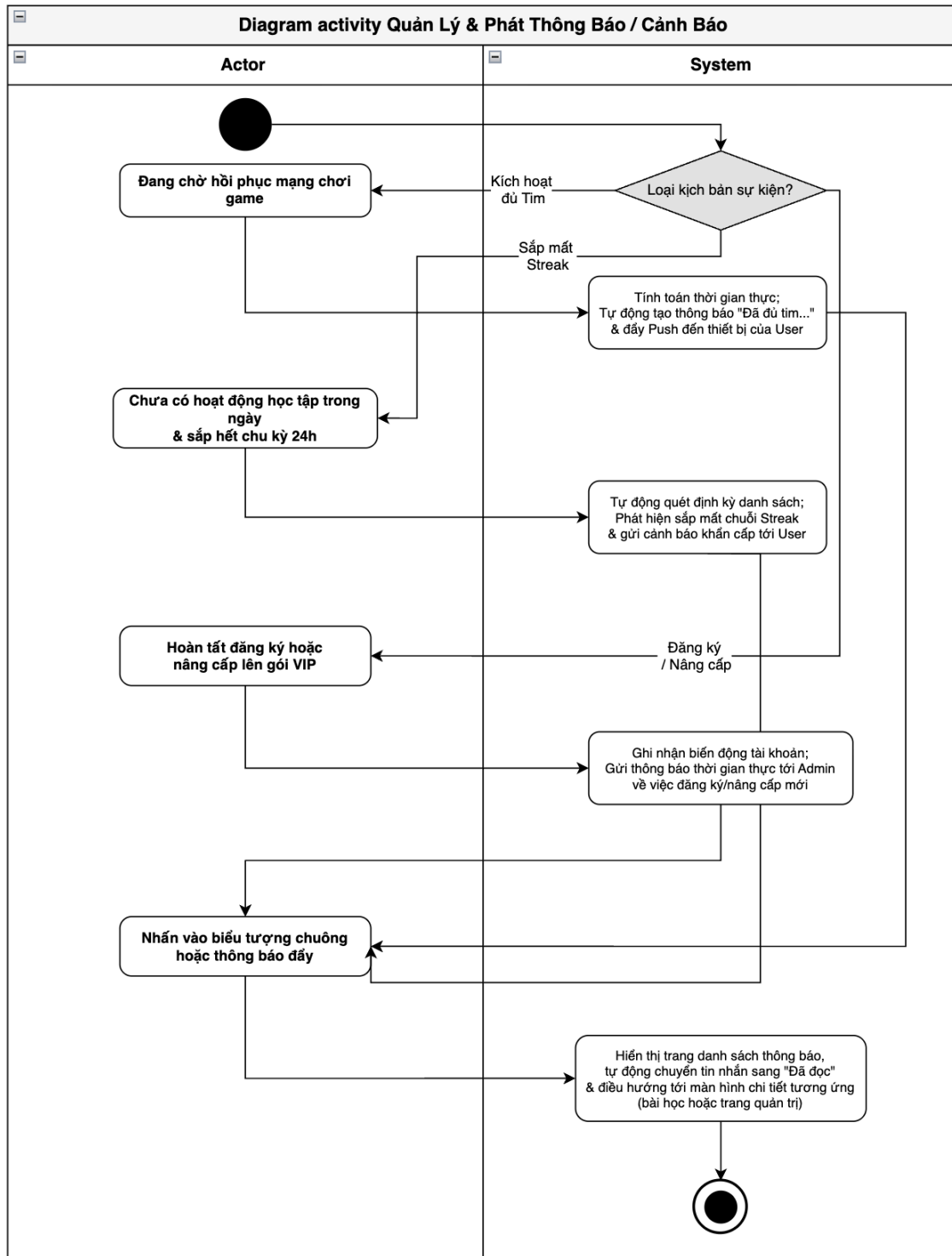
Hình 27: Activity Diagram
