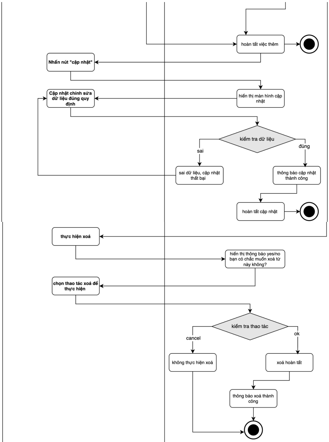
Hình 37: Activity Digram
