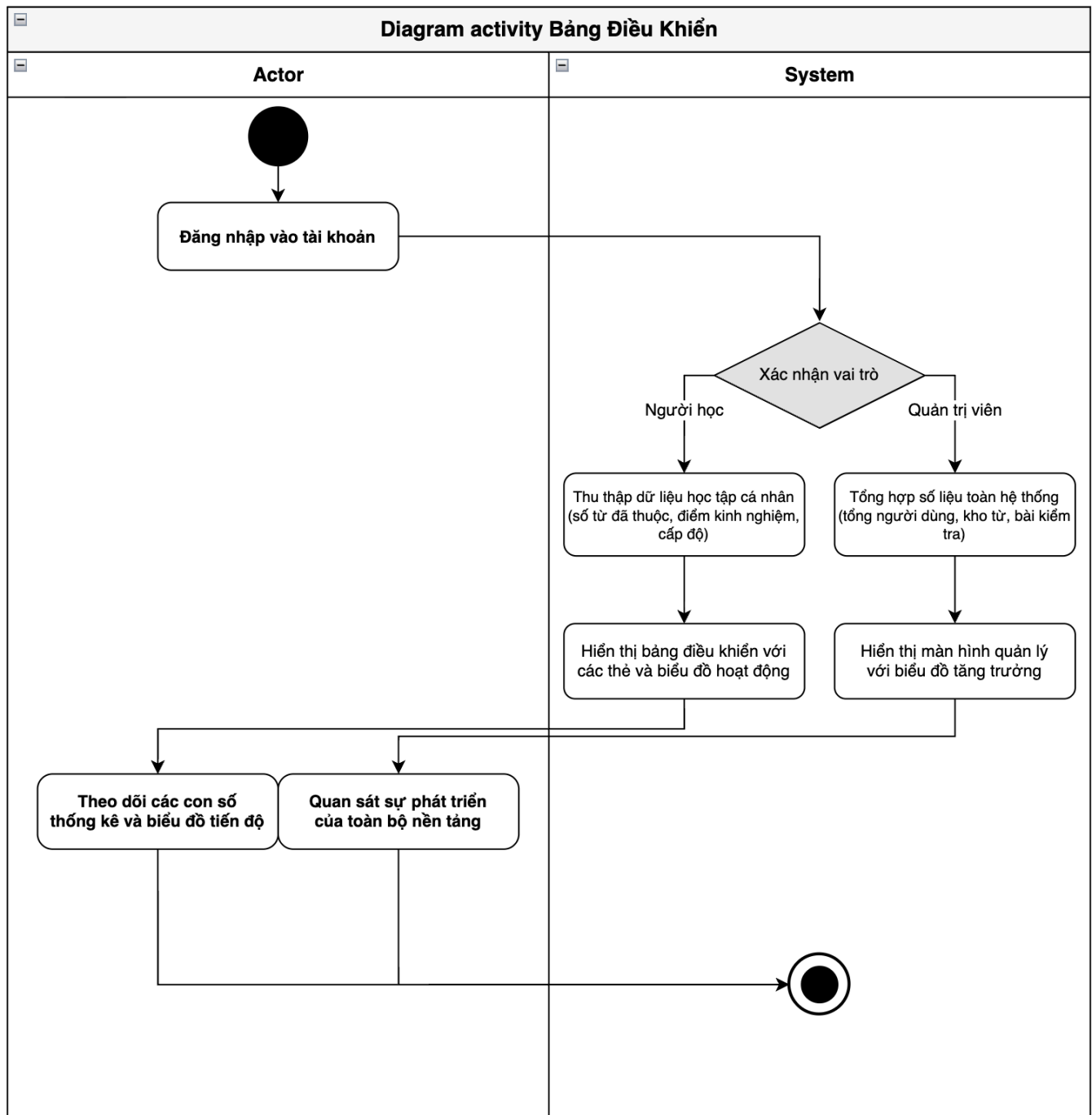
Hình 7:Activity Digram
