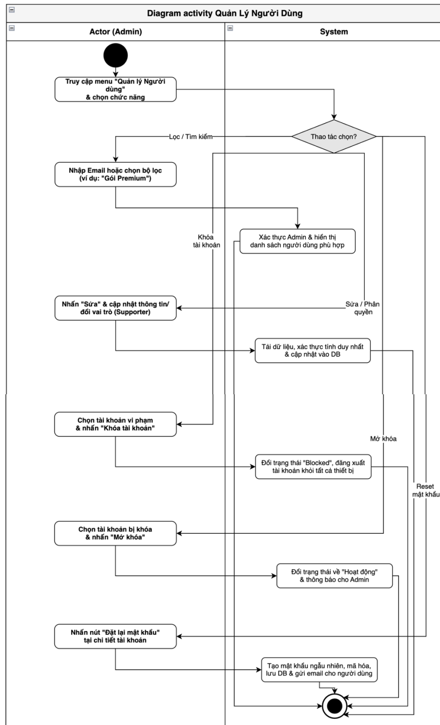
Hình 50: Activity Diagram
