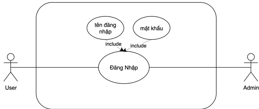
UC_Login
