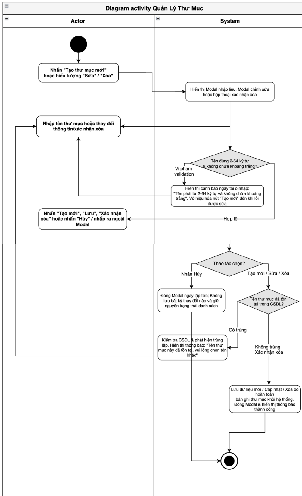
Hình 40: Activity Diagram
