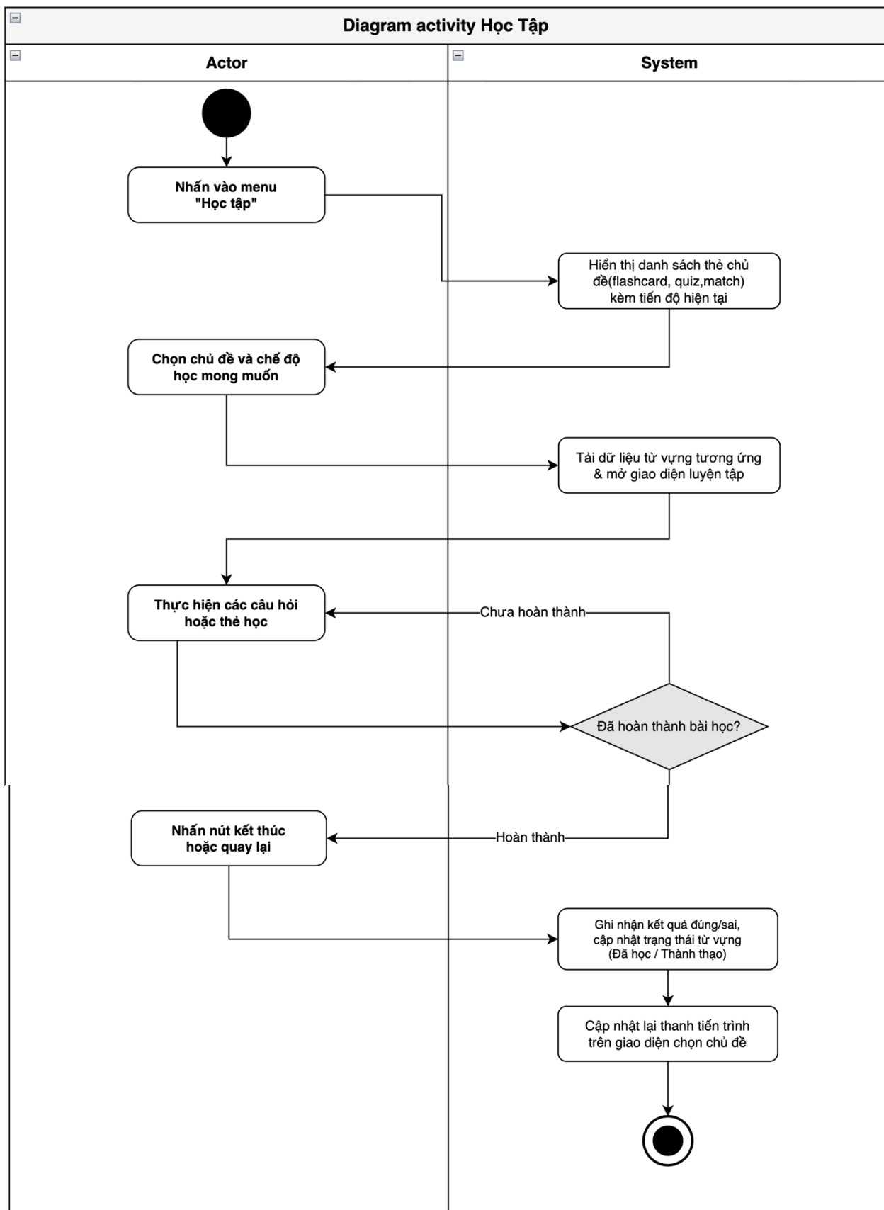
Hình 9: Activity Diagram
