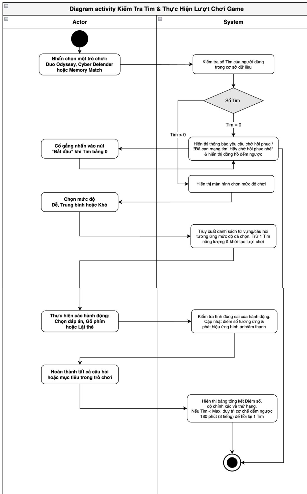
Hình 25: Activity Digram
