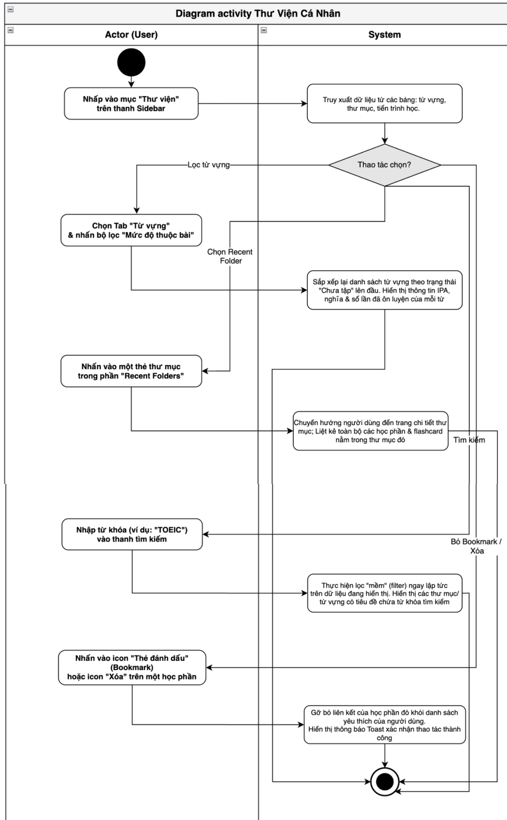
Hình 42: Activity Diagram
