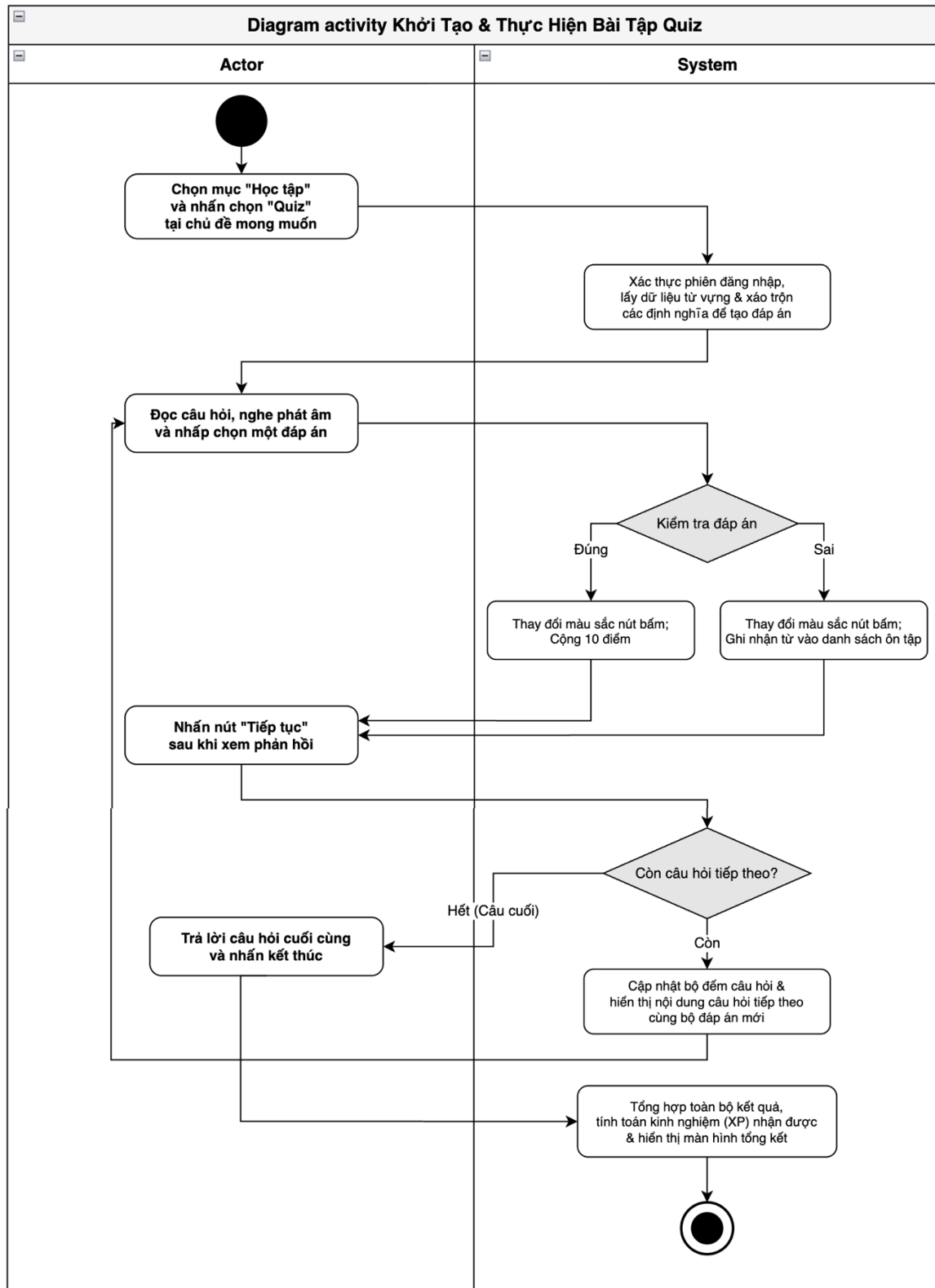
Hình 15: Activity Diagram
