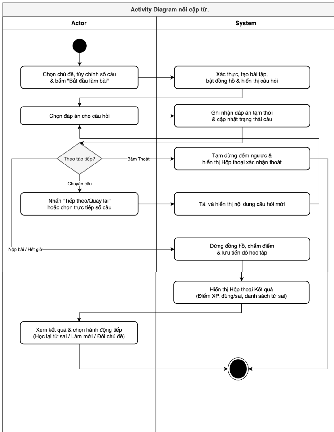
Hình 17: Activity Digram
