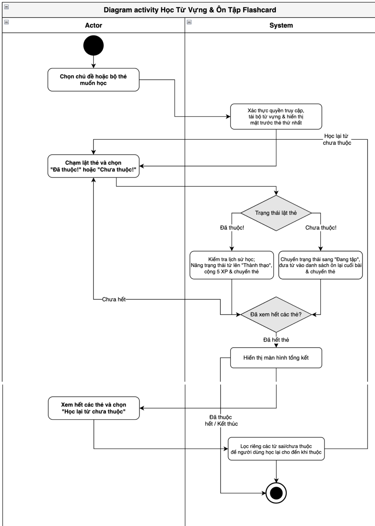
Hình 12: Activity Diagram
