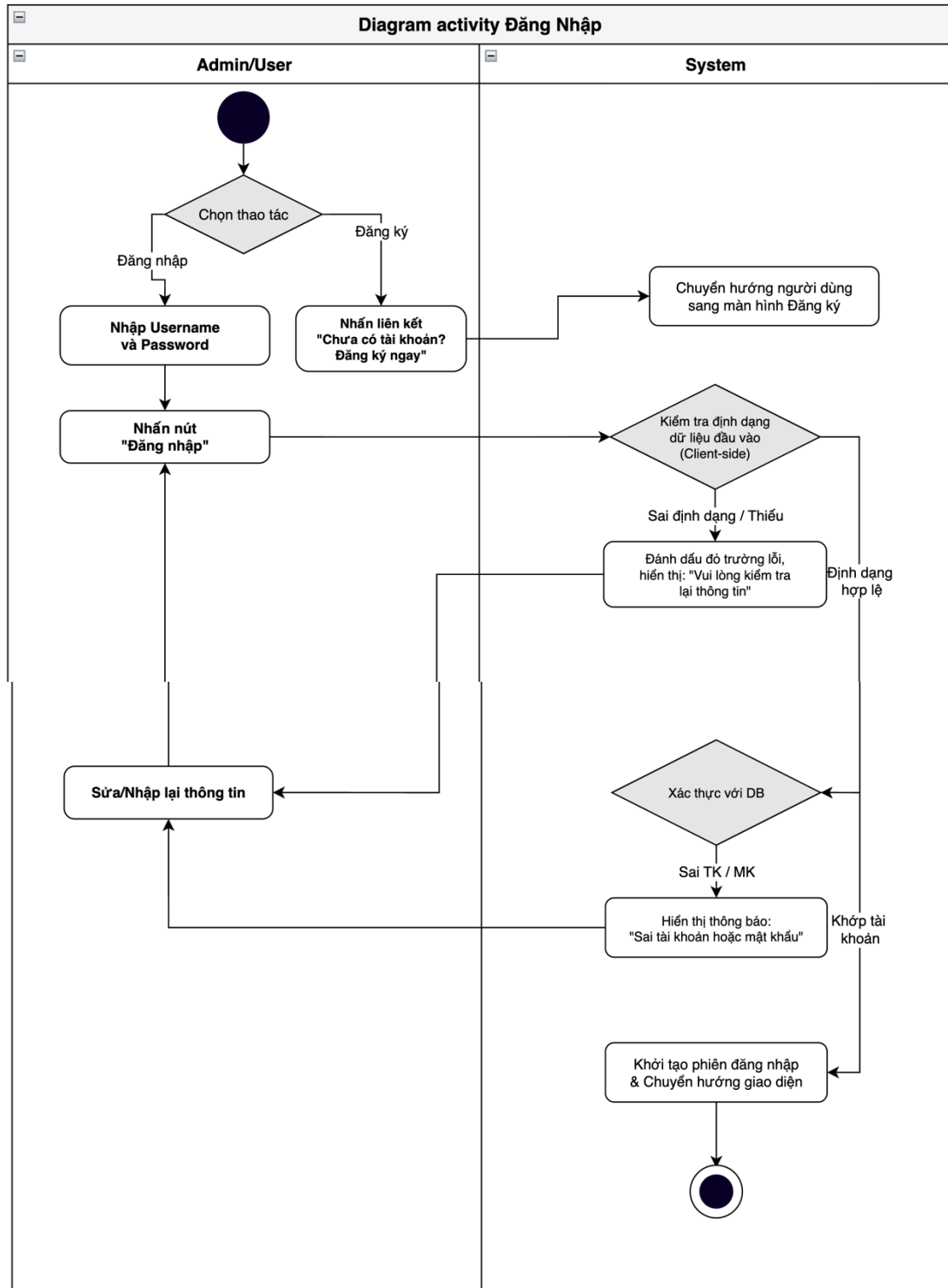
Hình 4:Activity Diagram
