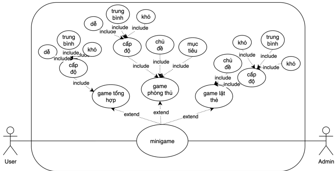
UC_Minigame.
