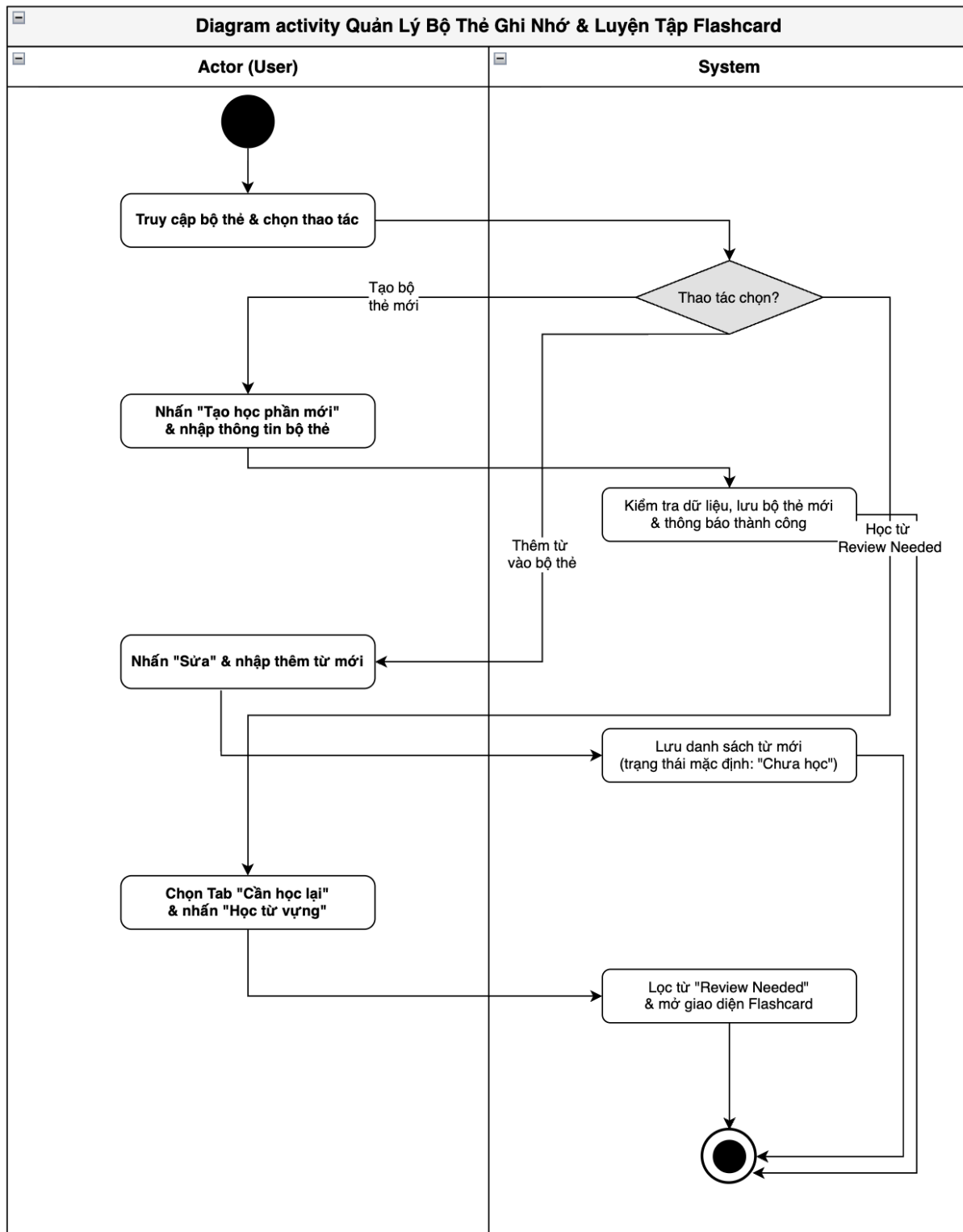
Hình 45: Activity Digram
