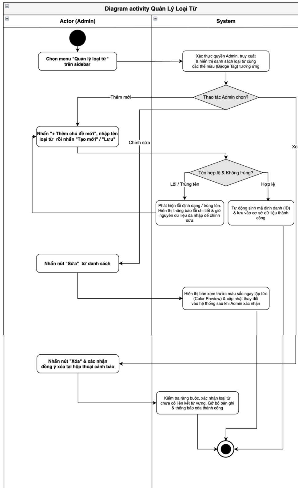
Hình 32: Activity Digram
